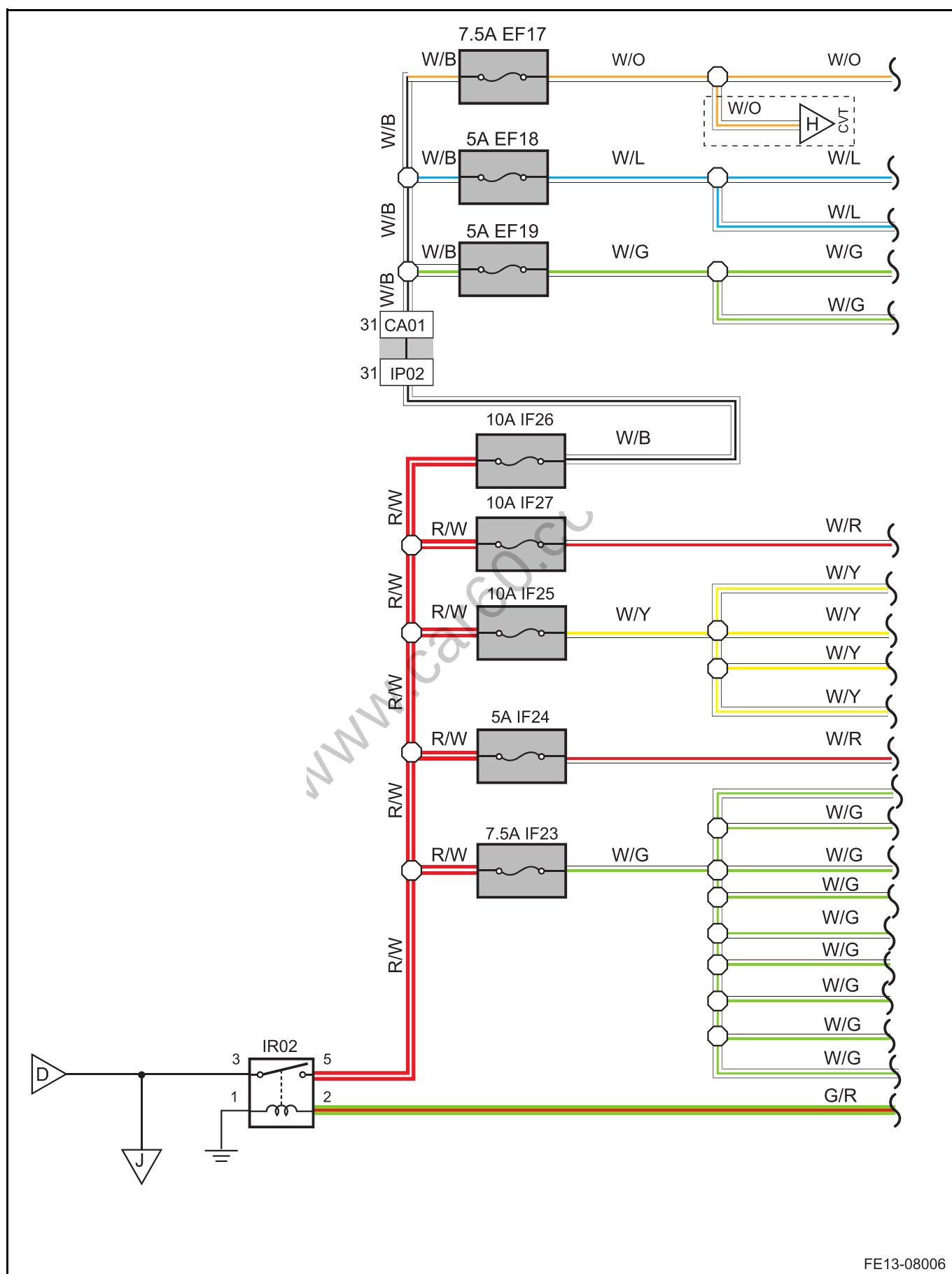
电源配电图 6
