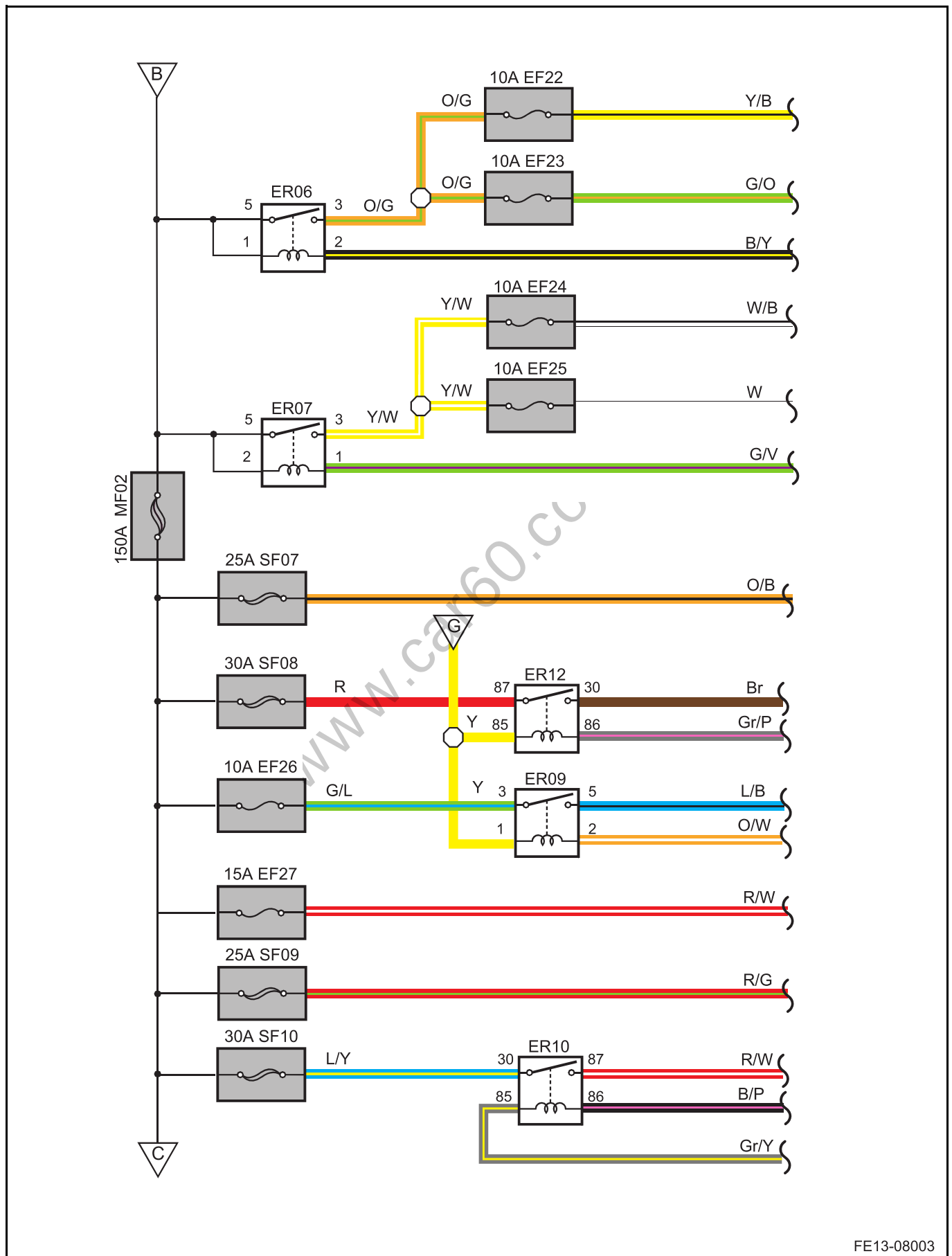
电源配电图 3
