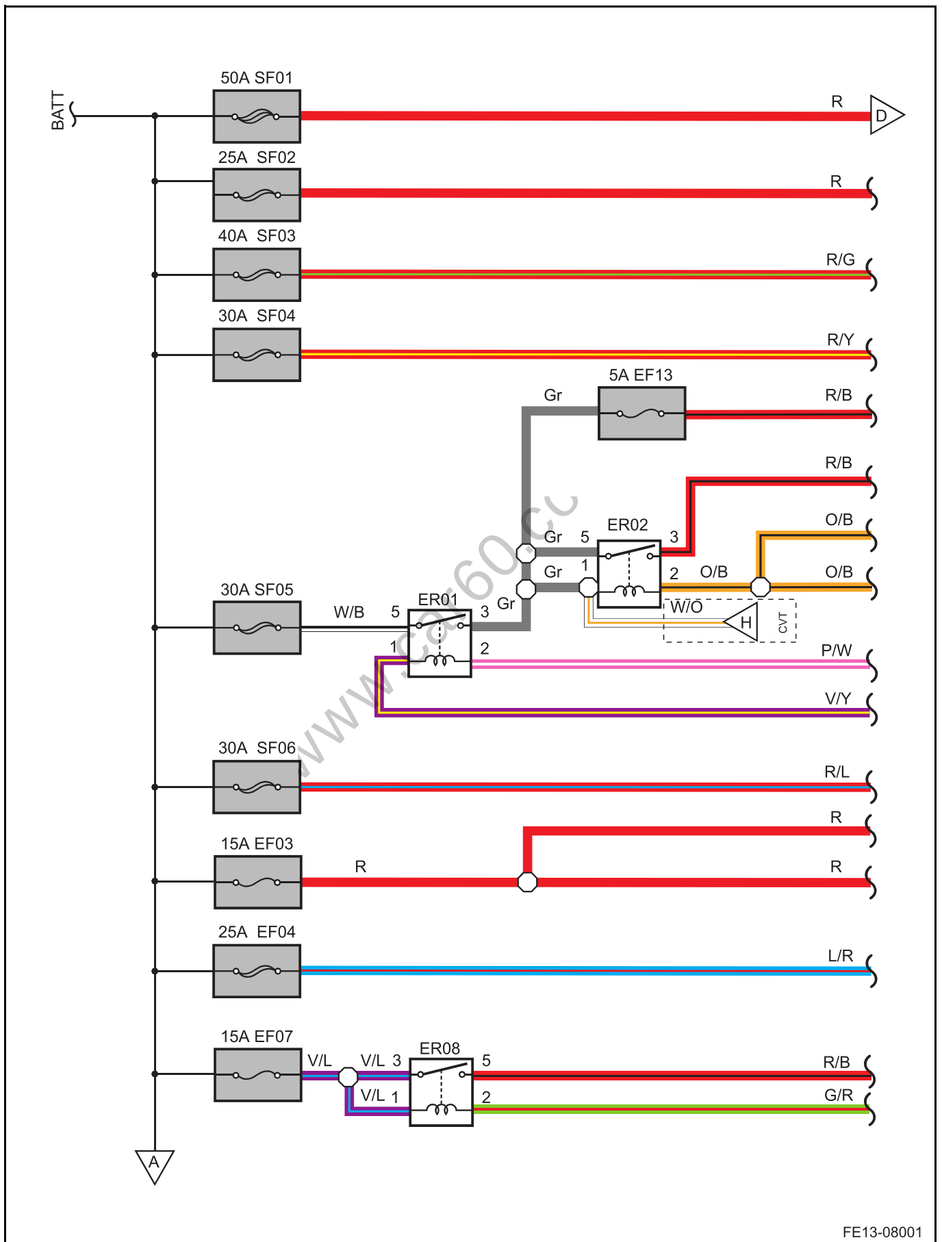
电源配电图 1
